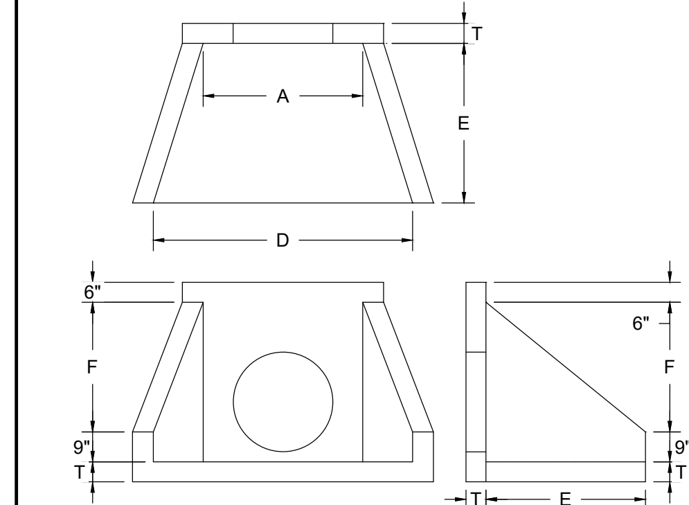
PRECAST CONCRETE HEADWALL N.T.S.
